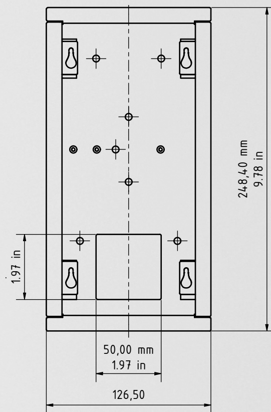
Unterputzgehäuse
